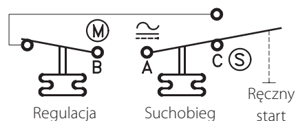
Schemat podłączenia
