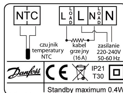
Schemat DEVlreg™ Smart
