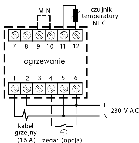
Schemat DEVlreg™ 316
