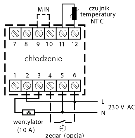
Schemat DEVlreg™ 316
