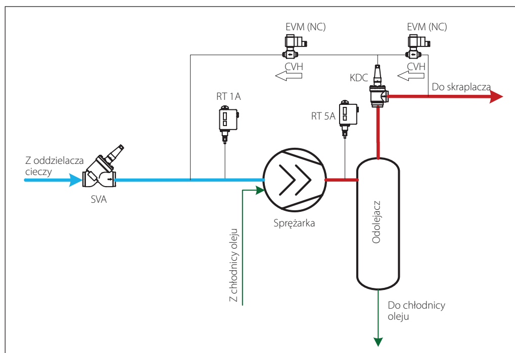
Przykład instalacji 6.2.3: Regulacja nadciśnienia oleju z zaworem KDC i pilotami EVM
