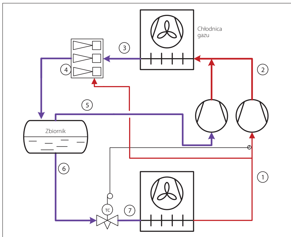
Rysunek 1.15: Transkrytyczny układ na CO 2 ze sprężaniem równoległym i eżeкторami parowymi
