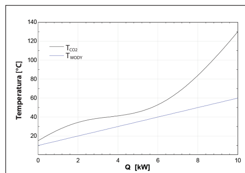
Rysunek 11.36: Odzysk ciepła z transkrytycznego obiegu CO 2
