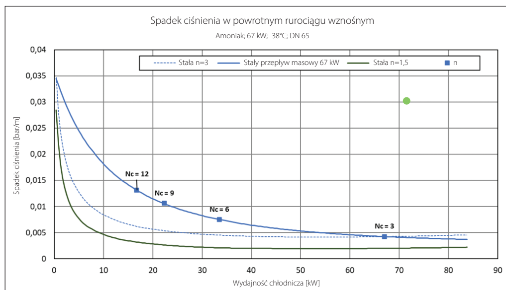
Rysunek 5.5.5: Spadek ciśnienia w powrotnym rurociągu wznoszącym przy obciążeniu częściowym
