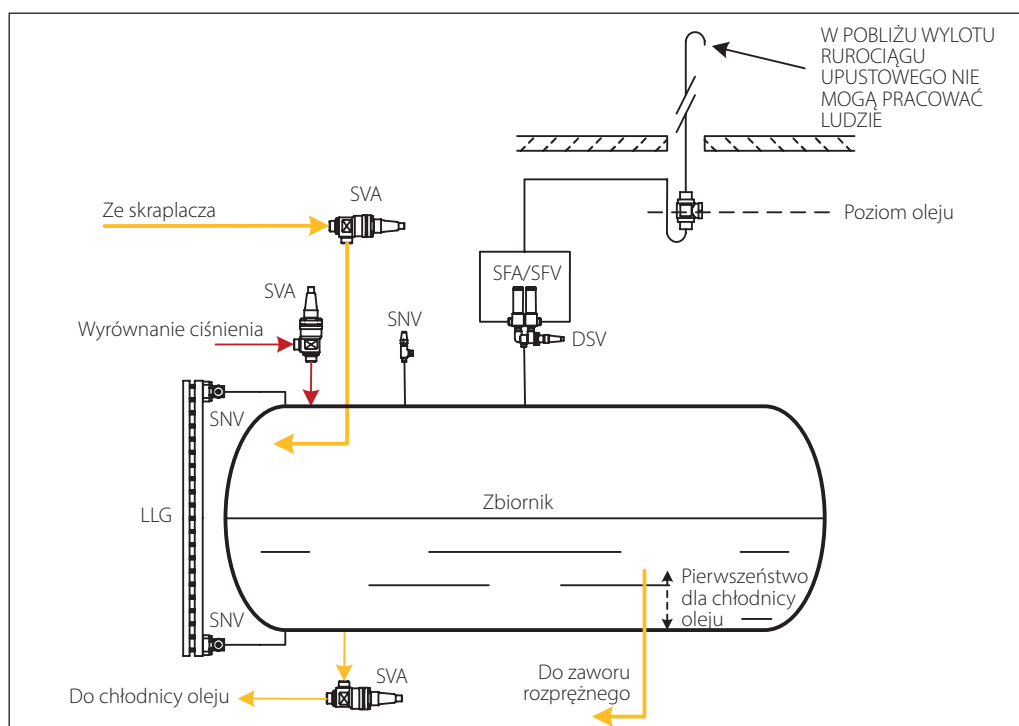
Przykład instalacji 7.1.1: Zawory bezpieczeństwa SFA + DSV
