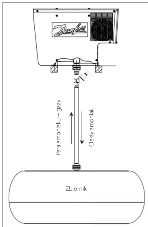
Rysunek 9.5: Odpowietrznacz Danfoss IPS podłączony do jednego punktu odpowietrzania
