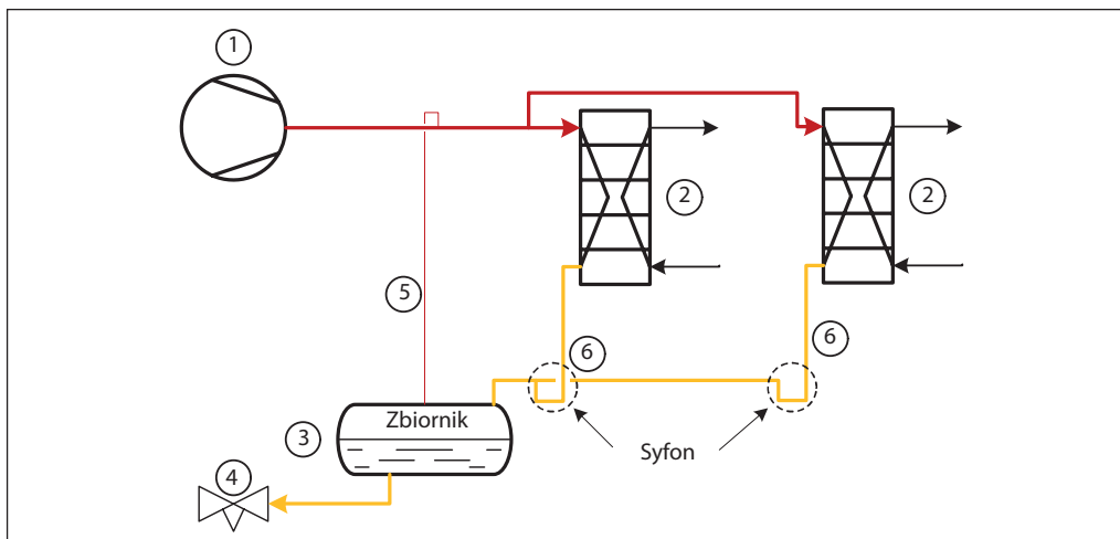
Rysunek 12.3.5: Układ z zaworem pływakowym niskiego ciśnienia i ze skraplaczami połączonymi równolegle
