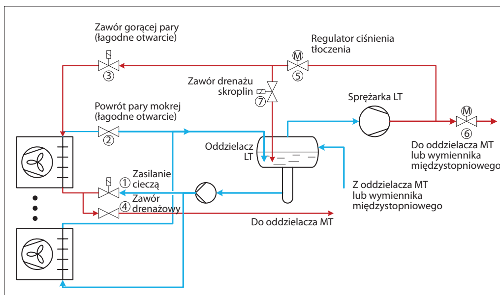
Rysunek 10.10.2: Schemat ideowy układu odszeraniania gorącą parą niskotemperaturowego parownika zasilanego pompowo, bez sprężarki do odszeraniania
