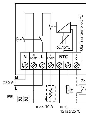
Schemat DEVIreg™ 530
