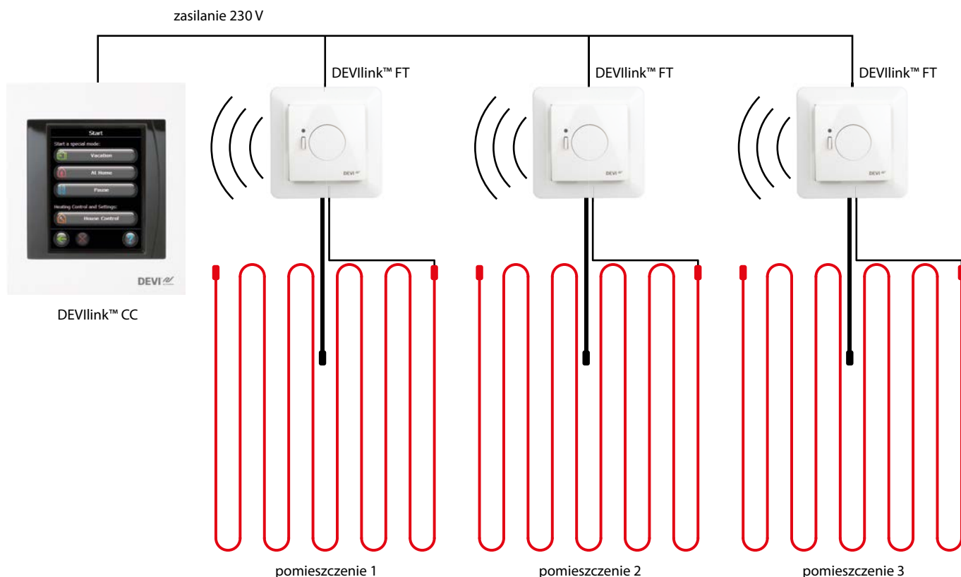
Schemat sterowania systemem akumulacyjnym w trzech pomieszczeniach z wykorzystaniem systemu DEVIlLink™
