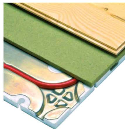
Widok warstw podłogi z ułożoną płytą DEVIcell Dry™
