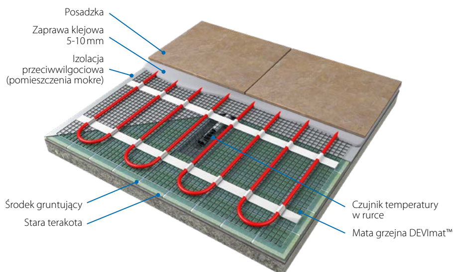
Podłoga cienkowarstwowa remontowana na starej terakocie
