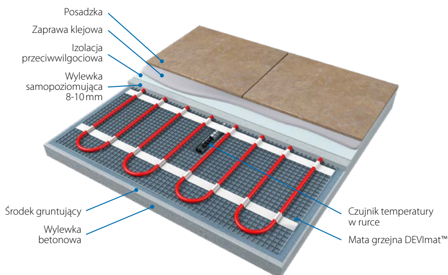
Podłoga cienkowarstwowa w kabinie natryskowej
