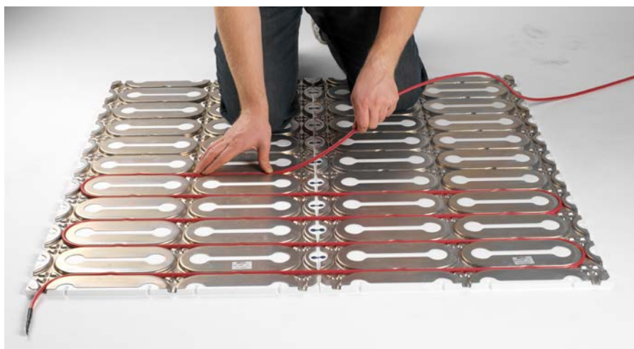
Sposób montażu kabla grzejnego z użyciem płyty DEVIcell Dry™
