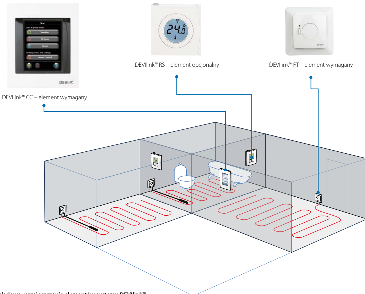
Przykładowe rozmieszczenie elementów systemu DEVlink™
