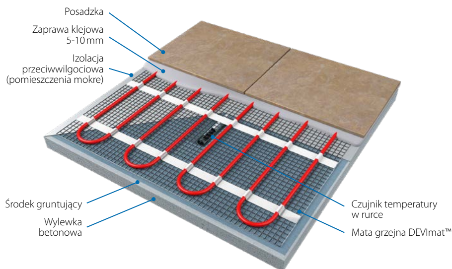
Podłoga cienkowarstwowa na nowej wylewce
