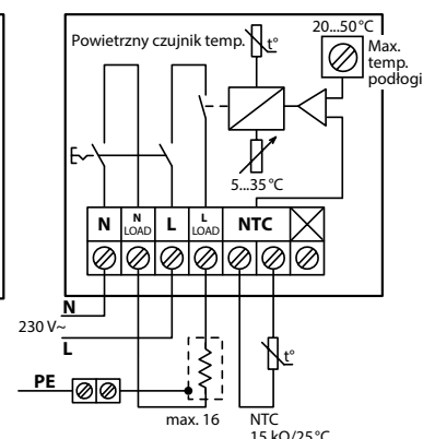
Schemat DEVIreg™ 532
