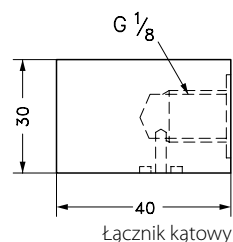
Łącznik kątowy
