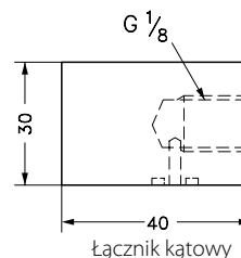
Łącznik kątowy
